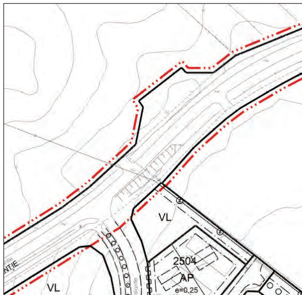
Kuva. Ote asemakaavaehdotuksesta, uusi liittymä.
