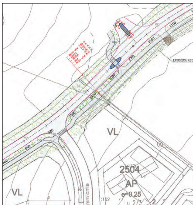
Kuva. Ote katusuunnittelmaluonnoksesta, uusi liittymä.
